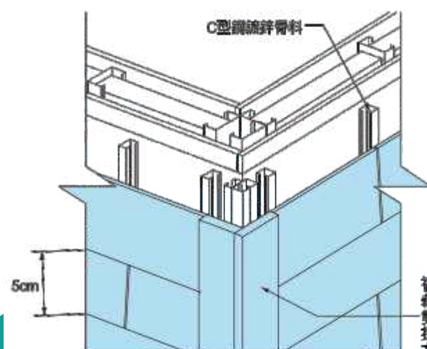
陽角交接示意圖
