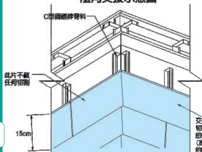
陰角交接示意圖
